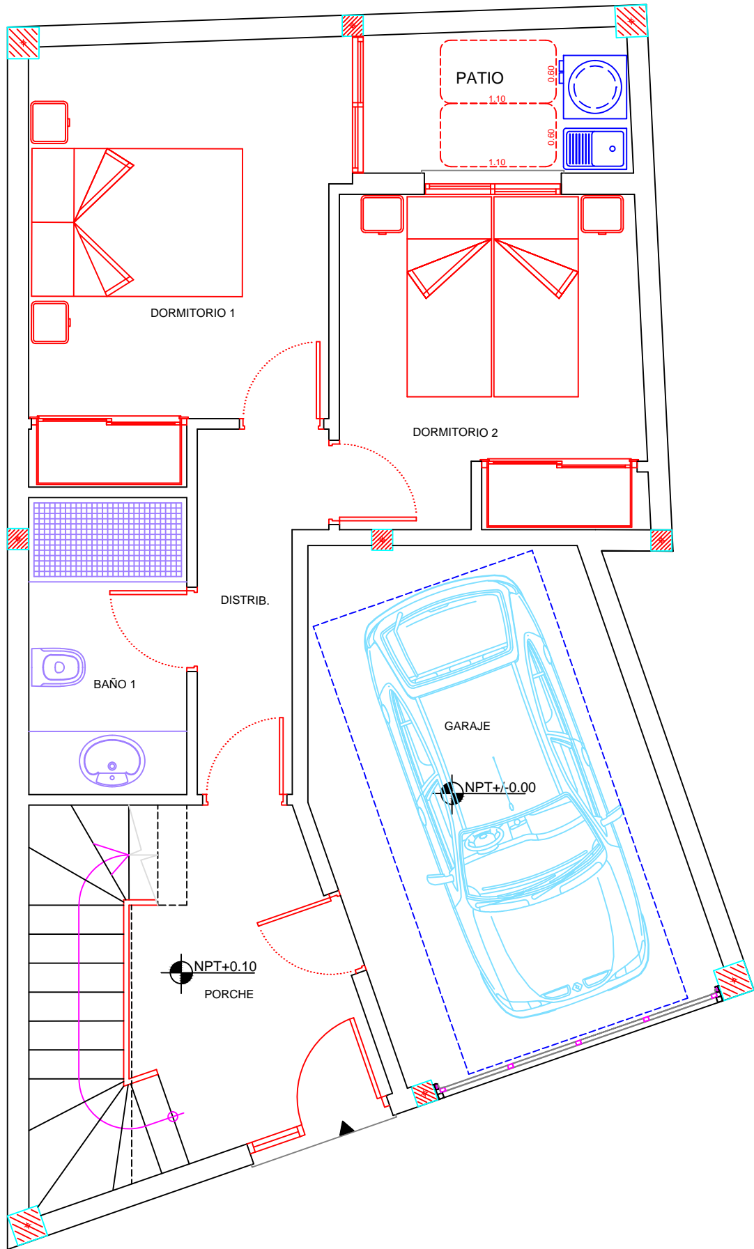
PLANTA BAJA
